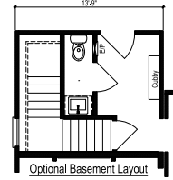
Optional Basement Layout
